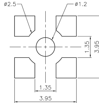
P.C.B. LAYOUT (印刷電路板配置)
